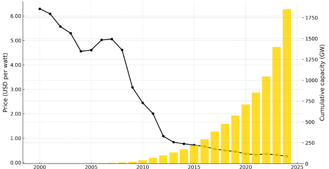
Solar PV module cost (constant 2024 US$ per watt)
